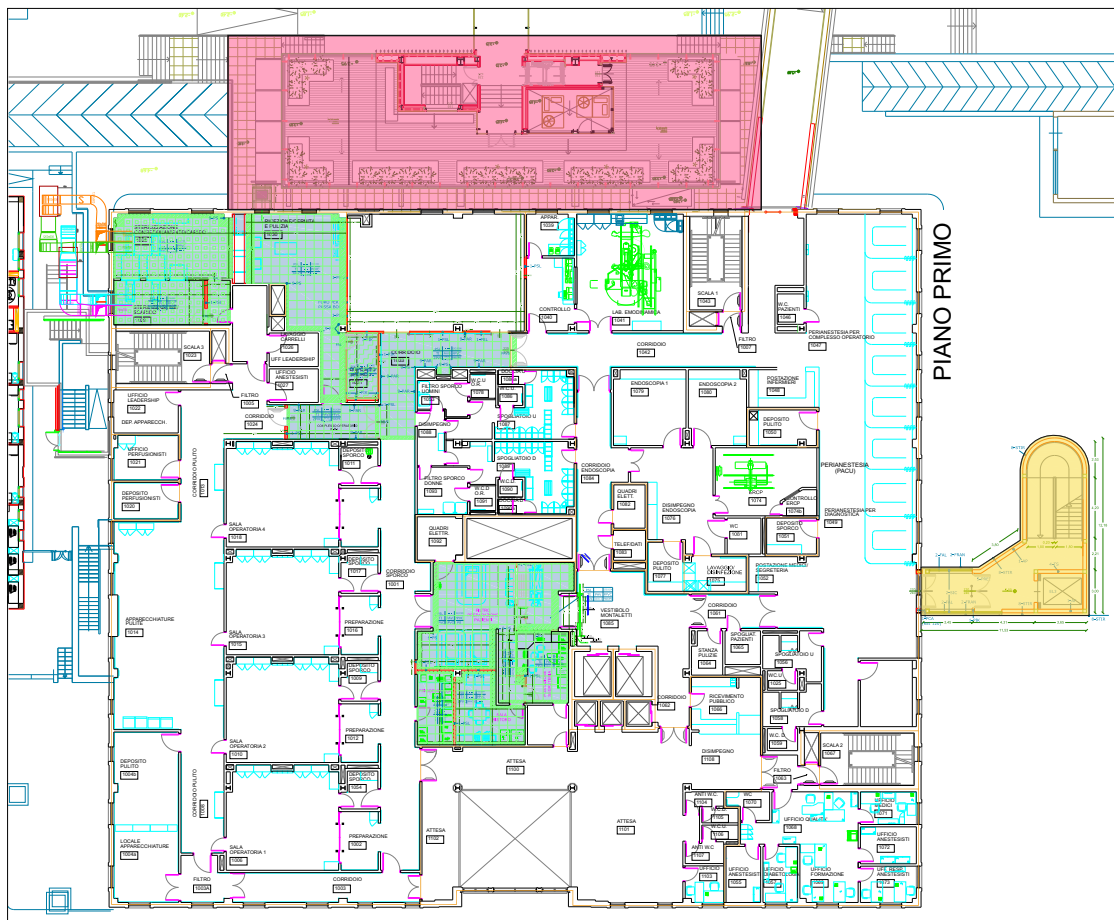
Planimetria Generale
